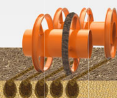
Двойной U-профильный каток DUW 580 мм
